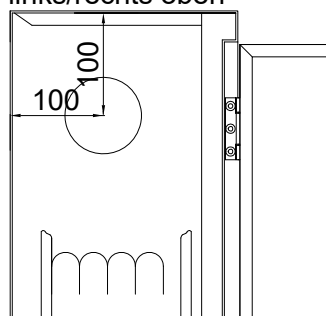
Detail Loch Feuerhahn links/rechts oben
