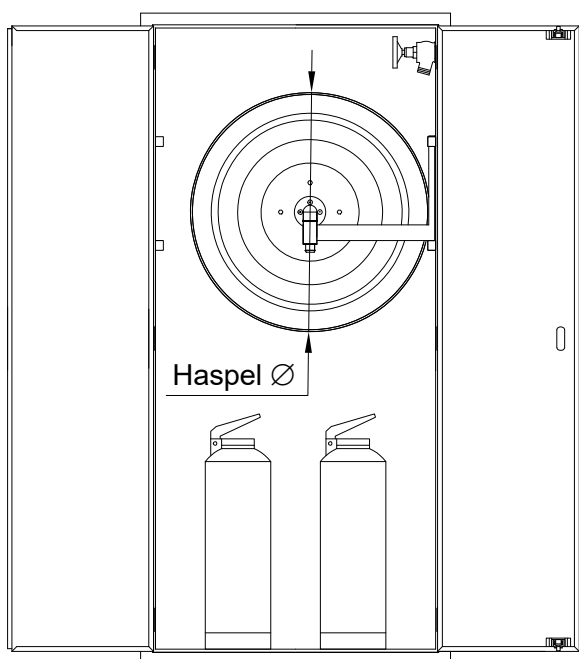
Befestigungspunkt Rückwand
